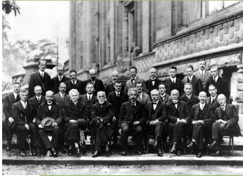
1927 tarihli resim uluslararası bir fizik konferansında çekilmiş. Ön sırada Albert Einstein ve gruptaki tek kadın Marie Curie görülüyor.
